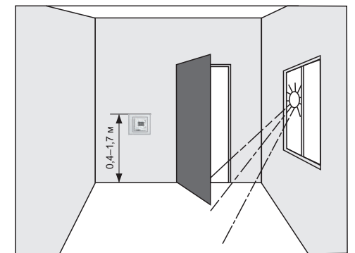
Рисунок 1. Монтаж терморегулятора і системи тепла підлога
