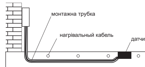
Рисунок 2. Спосіб монтажу датчика опадів при підігріві ґрунту
