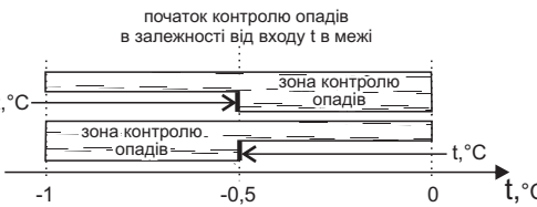
Рисунок 4. Мінімальні межі з гістерезисом > 1 °C.
