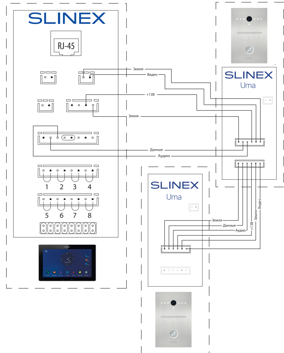
Схема 2. Подключение двух вызывных панелей.
