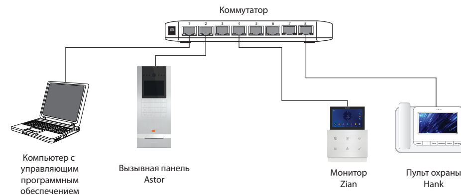
Схема 2. Пример подключения видеодомофона к локальной сети.
