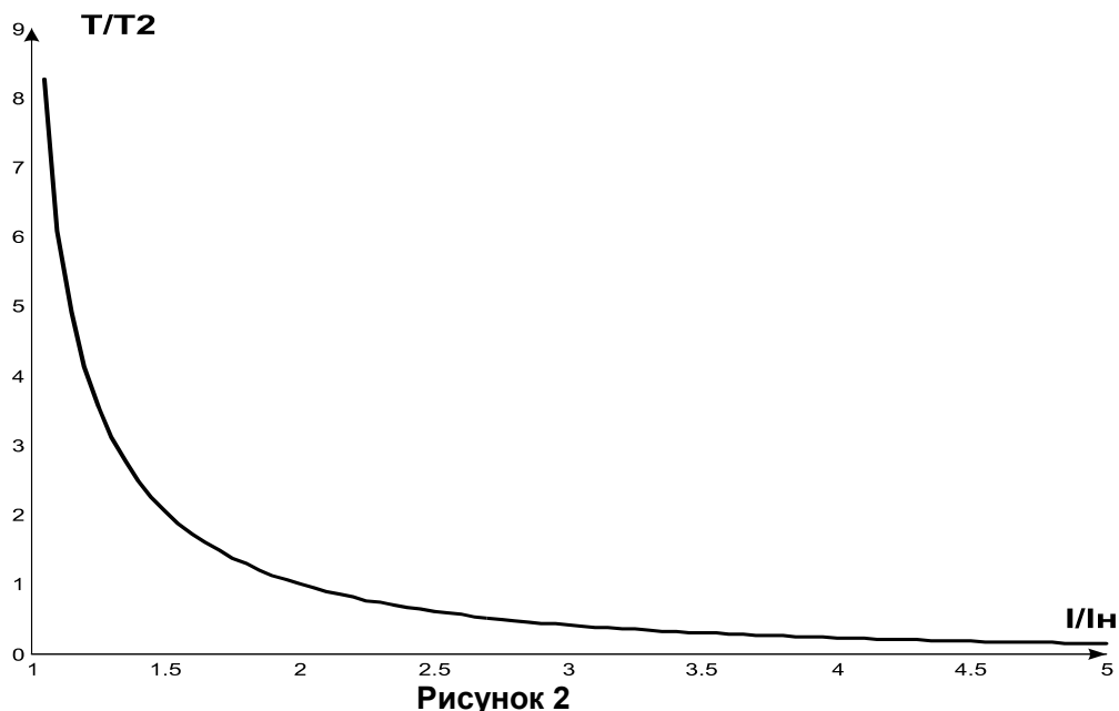
Струмо-часова характеристика
